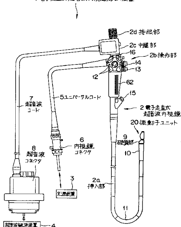
1 電子走査式超音波内視鏡診断装置
